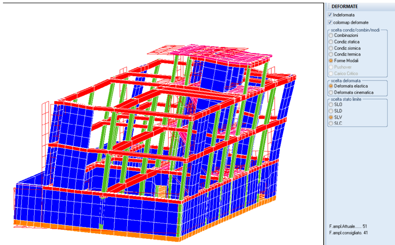
Fig.46-Primo modo di vibrare_Corpo A
