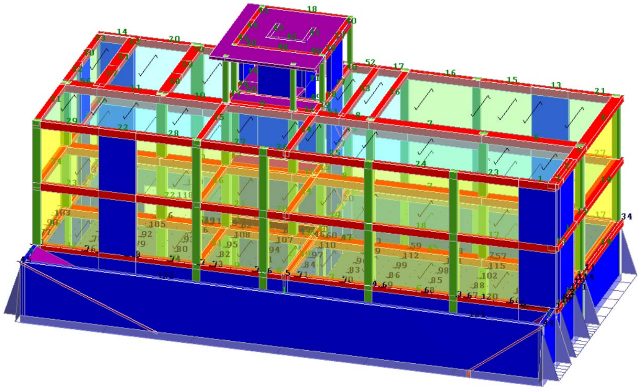
Fig.12-vista n.1_ 3D_Corpo A
