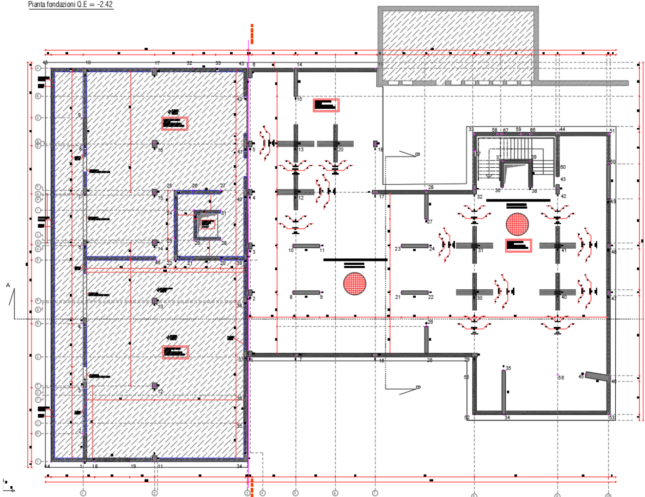
Figura 6 – Fondazioni corpo B FASE II
