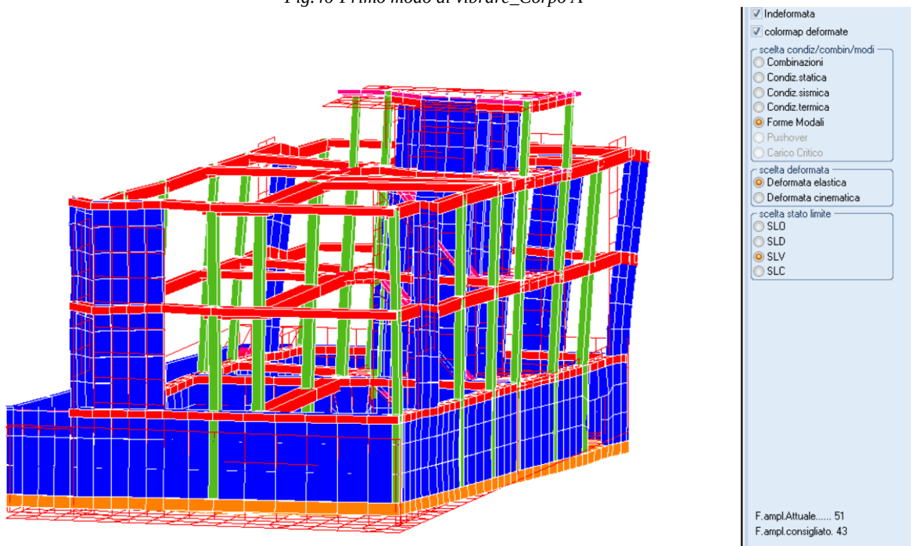
Fig.47-Secondo modo di vibrare_Corpo A
