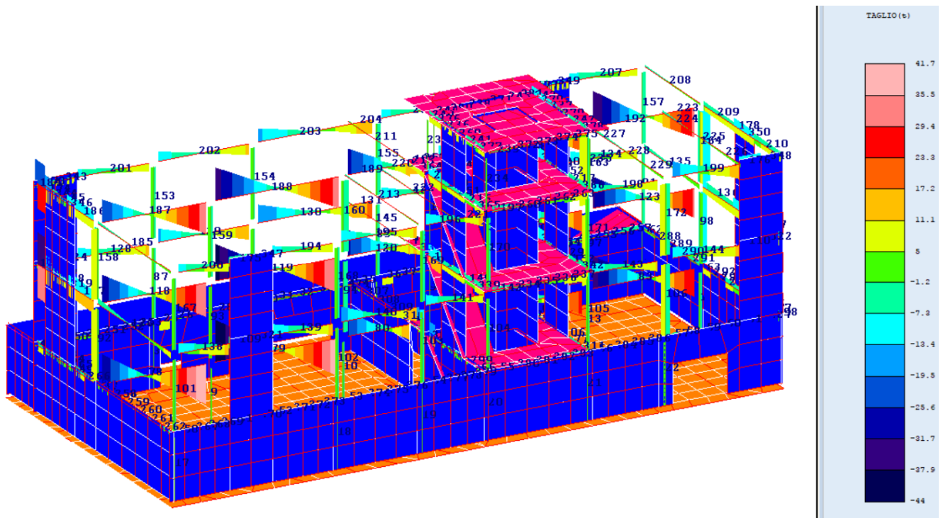
Fig.21-vista n.2_ Sforzi di Taglio Tx-Ty_involuppo_Corpo A
