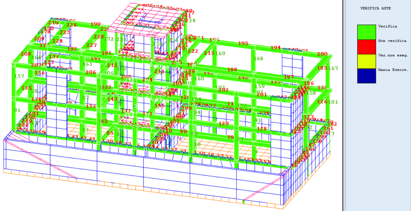
Fig.14-vista n.1_ Verifica aste in c.a. agli SLU-SLE_Corpo A
