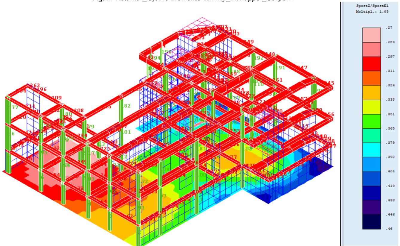
Fig.42-vista n.1_ Portanza_Corpo B
