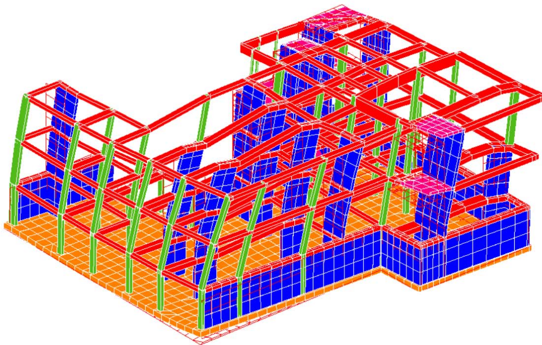
Fig.50-Secondo modo di vibrare_Corpo B
