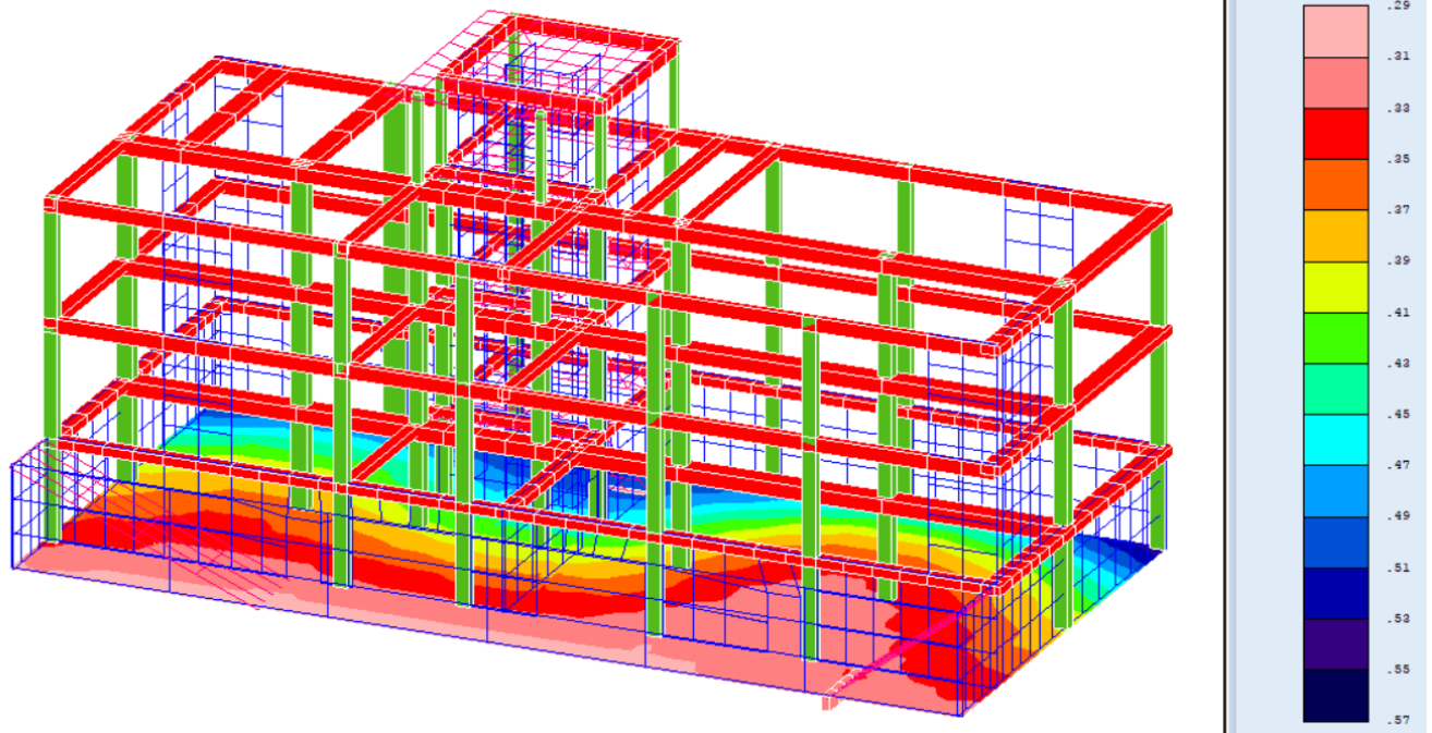
Fig.24-vista n.1_ Portanza_Corpo A
