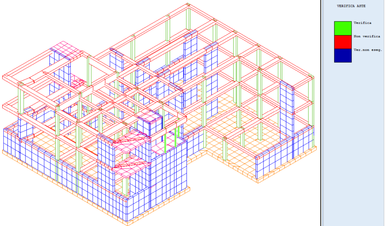
Fig.35-vista n.2_ Verifica aste in acciaio agli SLU-SLE _Corpo B
