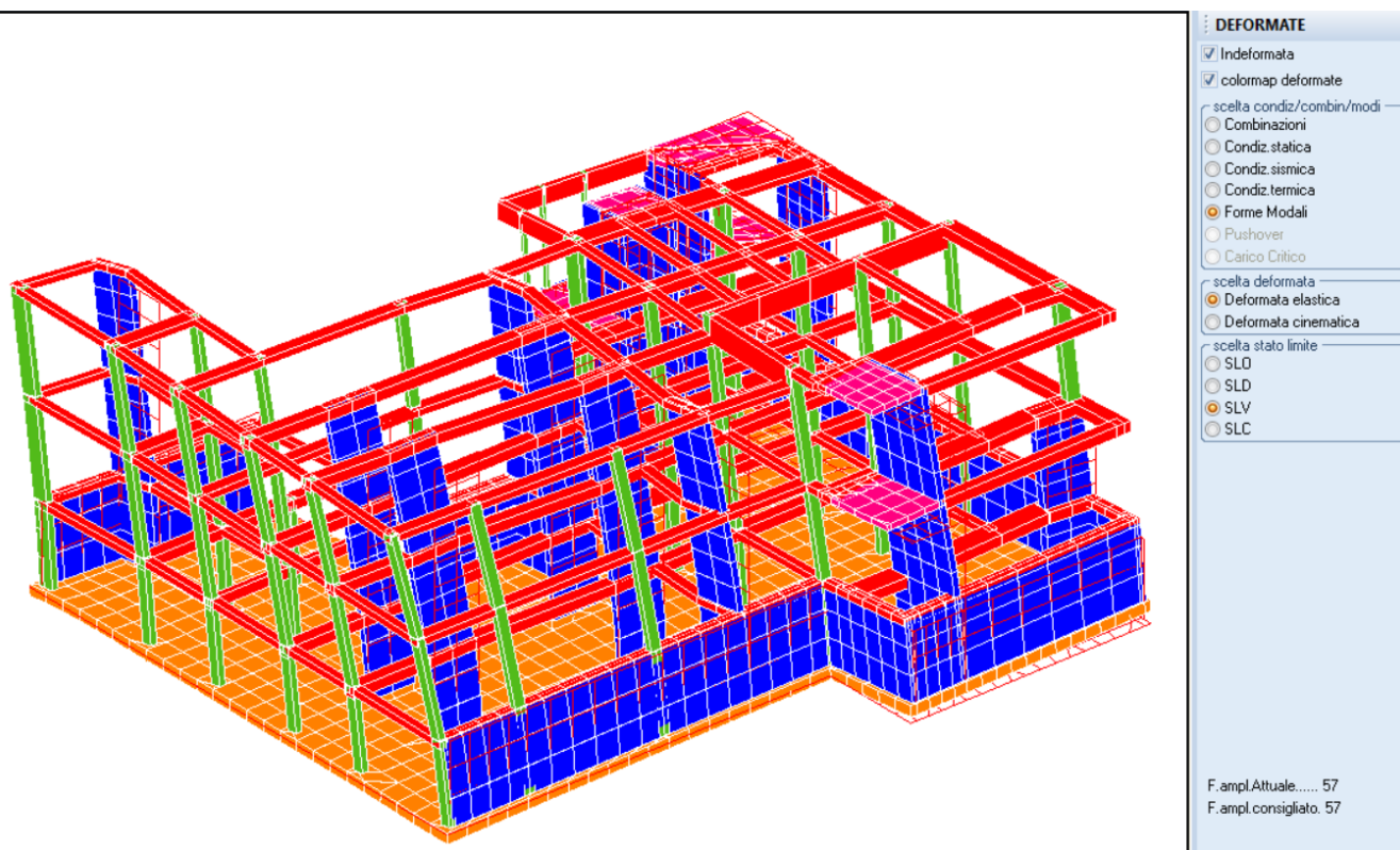
Fig.49-Primo modo di vibrare_Corpo B
