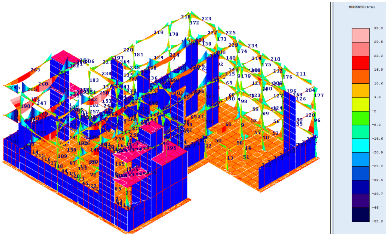
Fig.41-vista n.2_ Sforzo Momento Mx-My_involuppo _Corpo B
