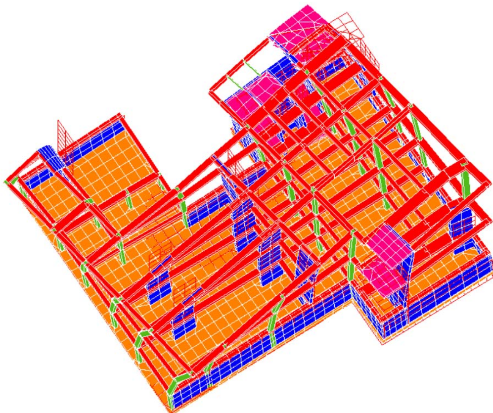
Fig.51-Terzo modo di vibrare_Corpo B
