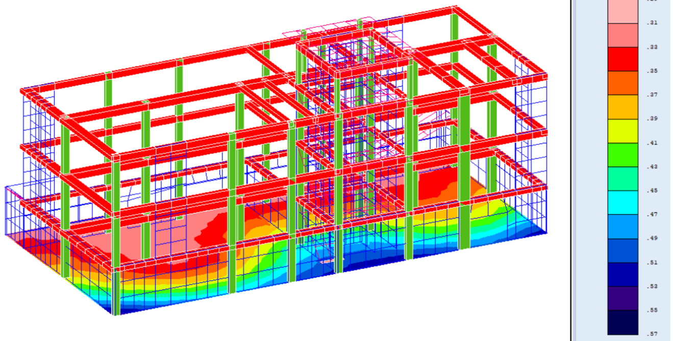
Fig.25-vista n.2_ Portanza_Corpo A
