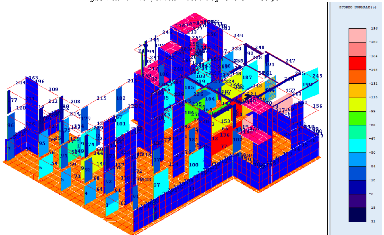
Fig.36-vista n.1_ Sforzo Normale N_involuppo _Corpo B
