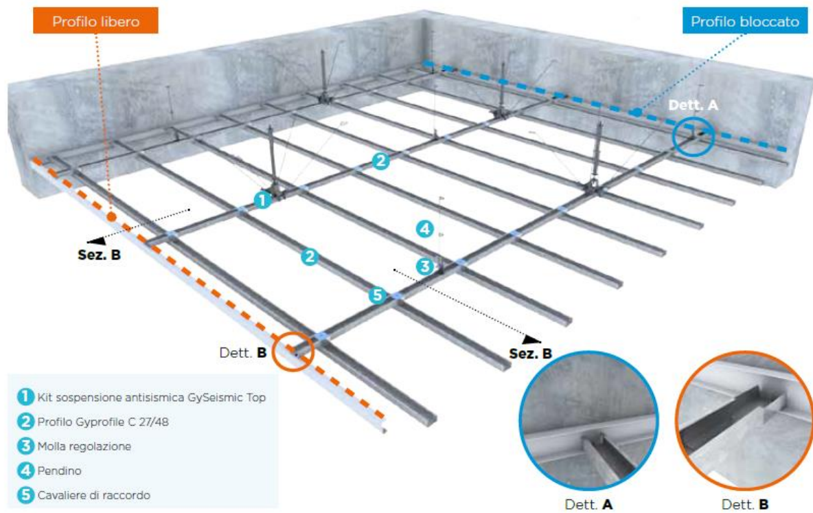
Fig. 2 - Installazione del sistema G-Seismic Top su controsoffitto in cartongesso continuo con doppia orditura metallica
