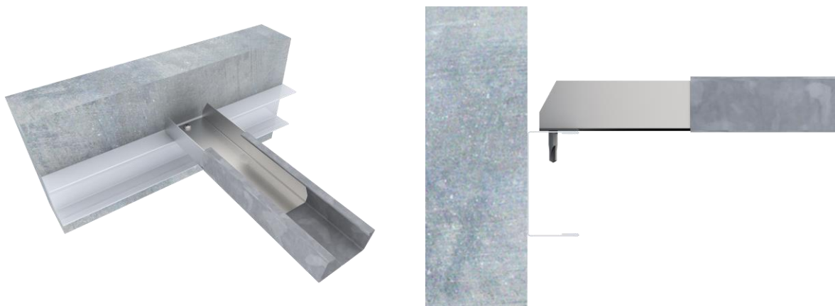
Fig. 3- Fissaggio dell'accessorio su profilo perimetrale con vite - VINCOLO CONDIZIONATO
