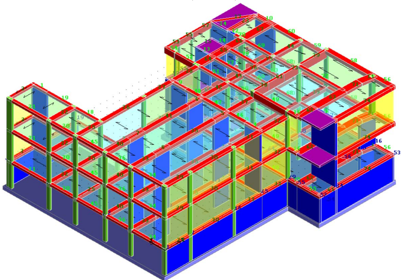
Fig.28-vista n.1_ 3D_Corpo B
