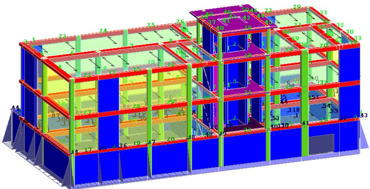
Fig.13-vista n.2_ 3D_Corpo A
