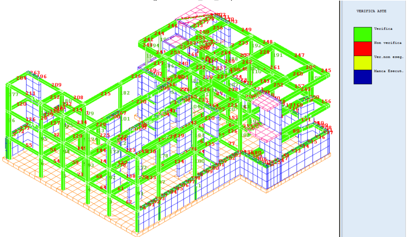
Fig.30-vista n.1_ Verifica aste in c.a. agli SLU-SLE_Corpo B
