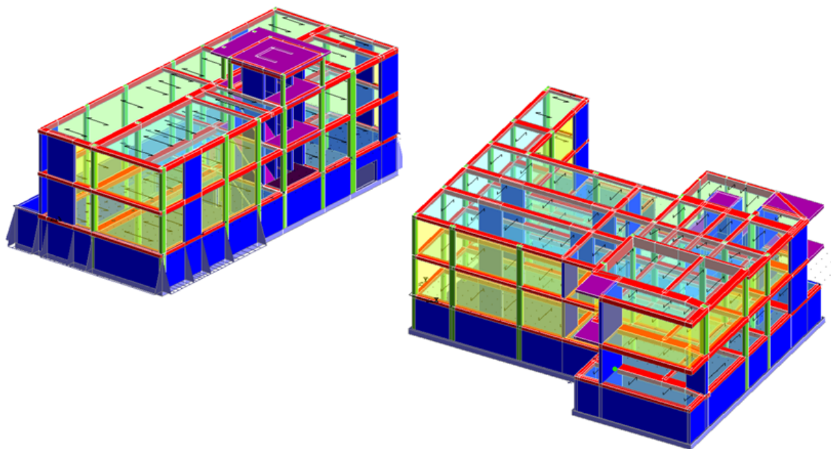
Figura 11 – Vista 3D corpo A e corpo B
