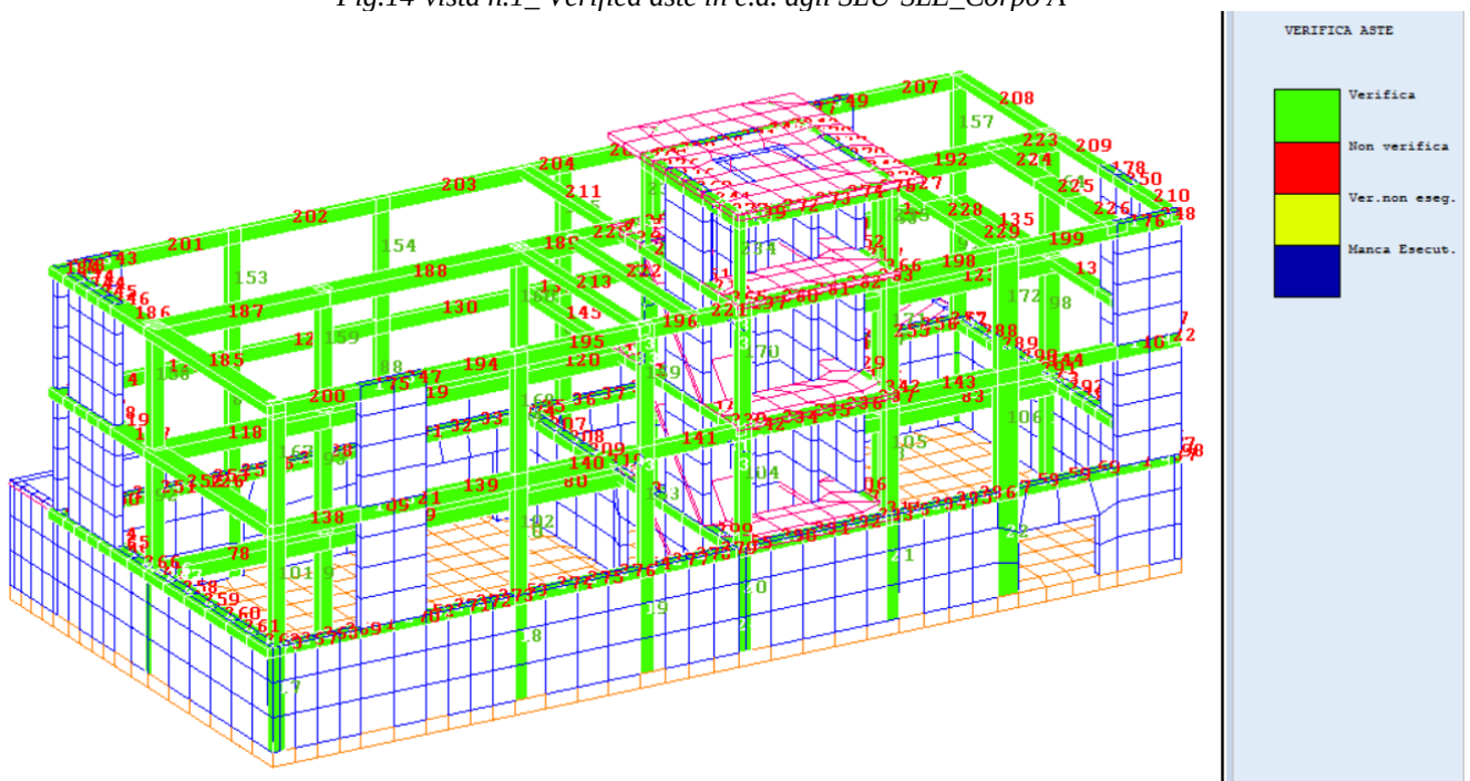
Fig.15-vista n.2_ Verifica aste in c.a. agli SLU-SLE_Corpo A
