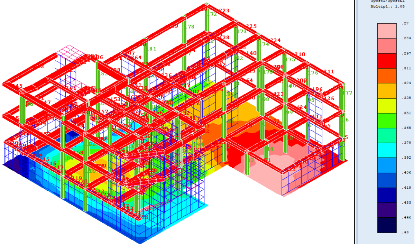
Fig.43-vista n.2_ Portanza_Corpo B
