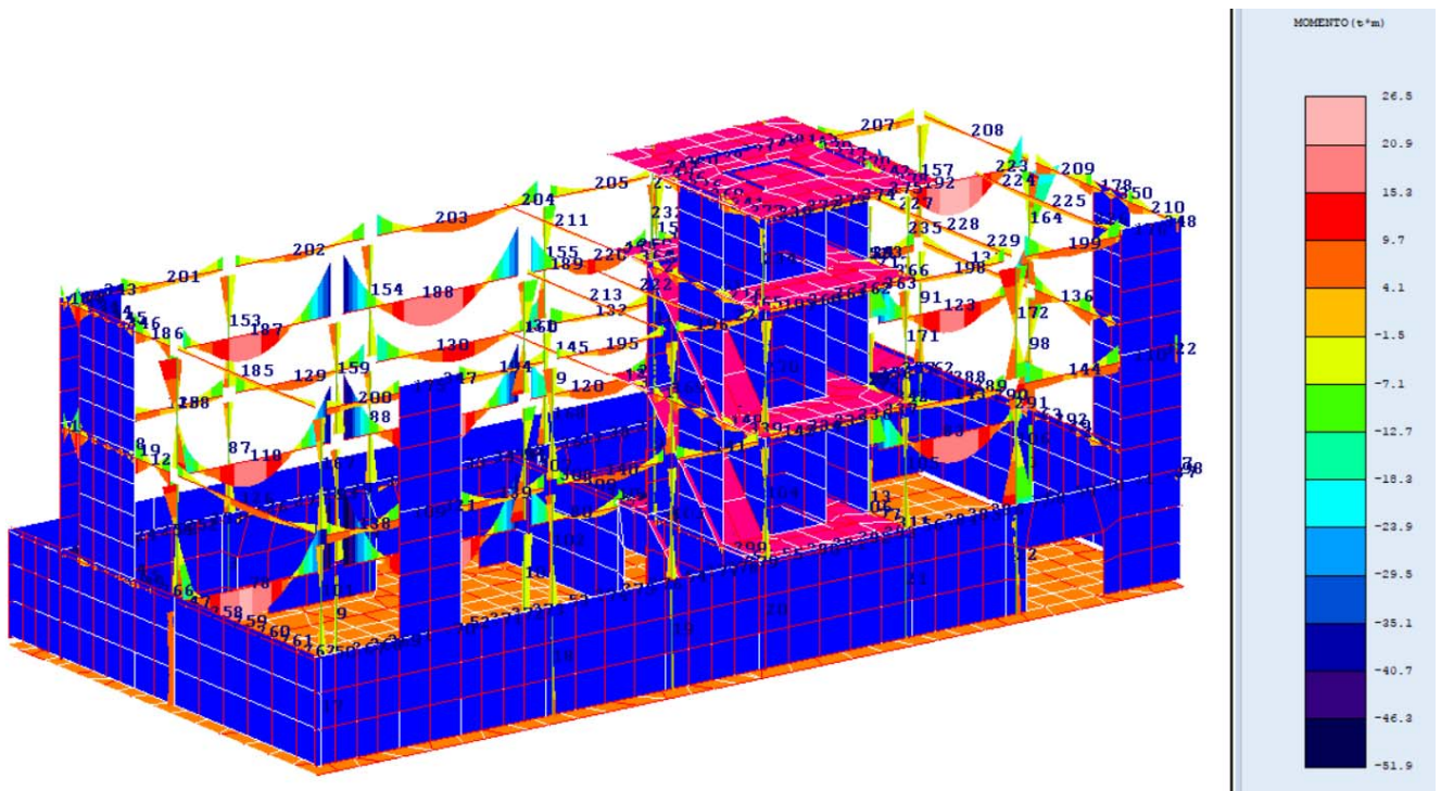
Fig.23-vista n.2_ Sforzi Momento Mx-My_involuppo_Corpo A
