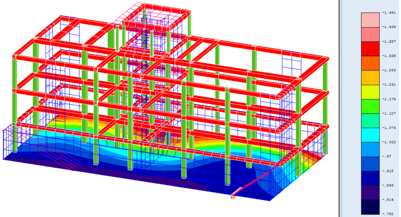
Fig.26-vista n.1_ Spostamenti z_Corpo A
