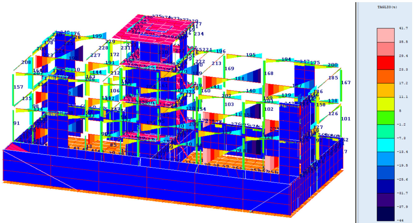
Fig.20-vista n.1_ Sforzi di Taglio Tx-Ty_involuppo_Corpo A
