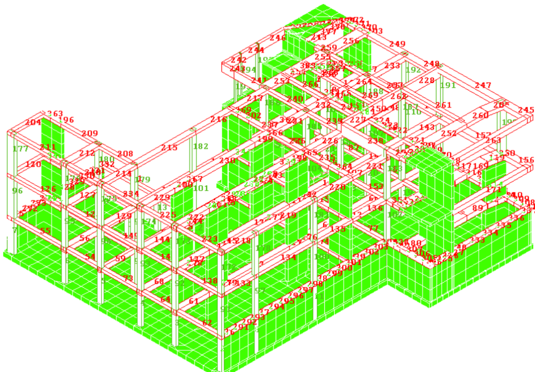
Fig.32-vista n.1_ Verifica shell in c.a. agli SLU-SLE _Corpo B
