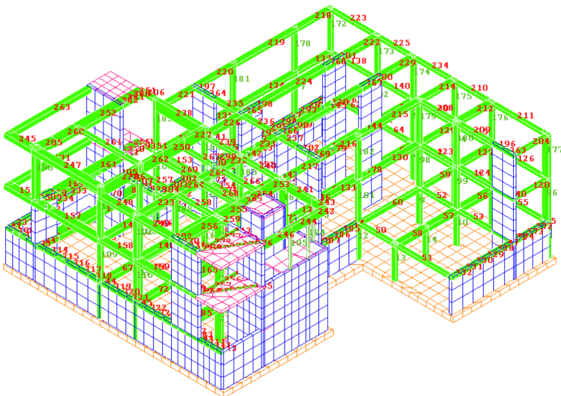
Fig.31-vista n.2_ Verifica aste in c.a. agli SLU-SLE _Corpo B
