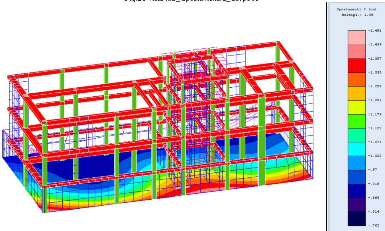
Fig.27-vista n.2_ Spostamenti z_Corpo A
