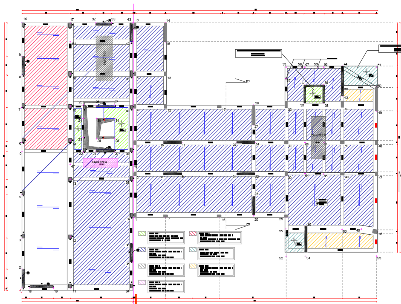
Figura 10 - Key plan Copertura
