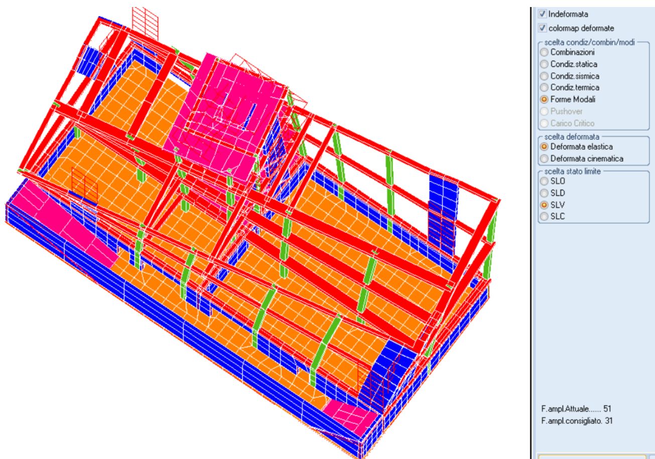
Fig.48-Terzo modo di vibrare_Corpo A
