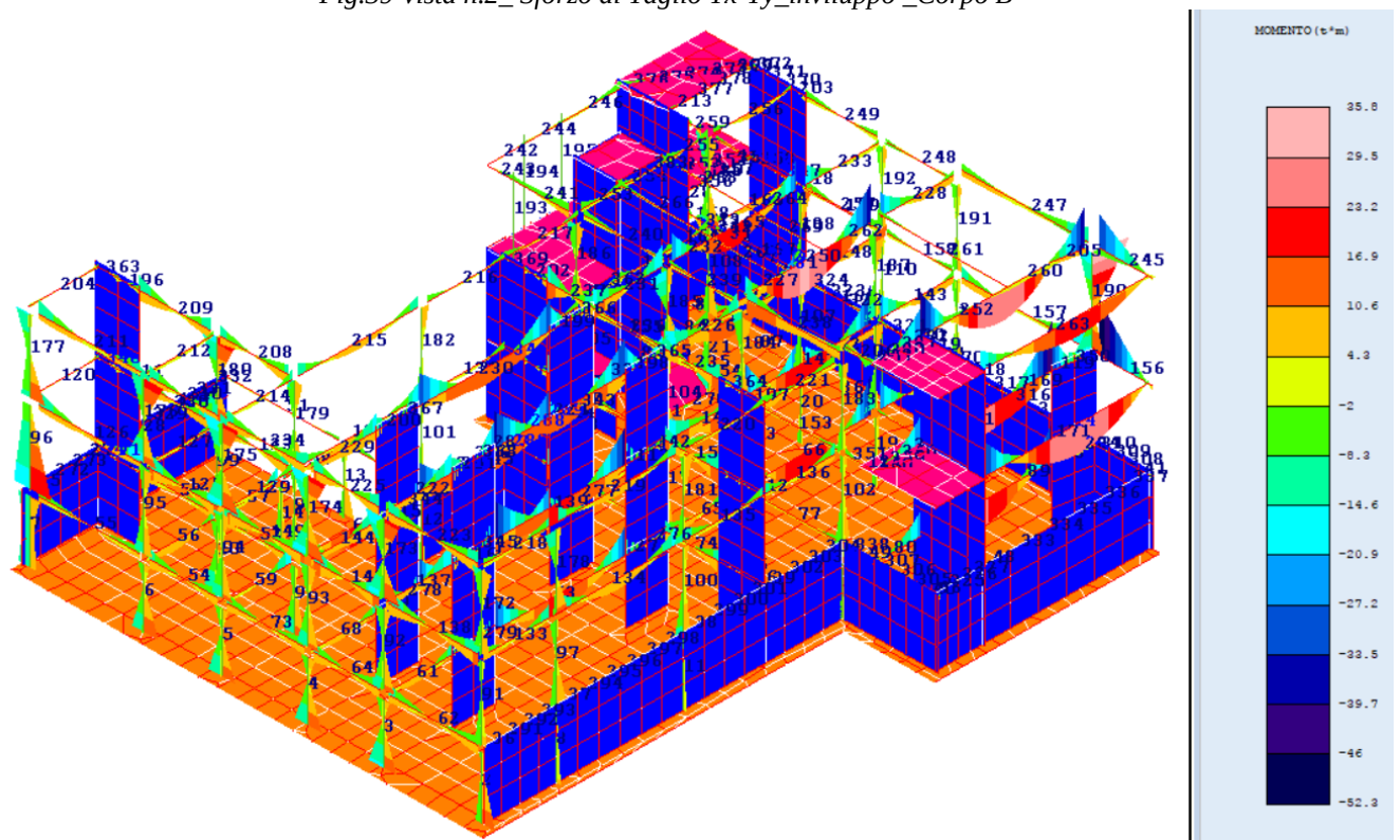
Fig.40-vista n.1_ Sforzo Momento Mx-My_involuppo _Corpo B
