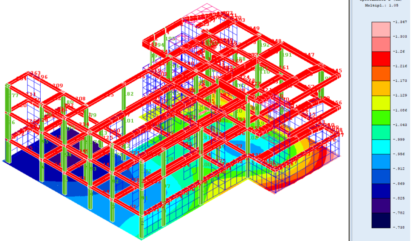
Fig.44-vista n.1_ Spostamenti z_Corpo B
