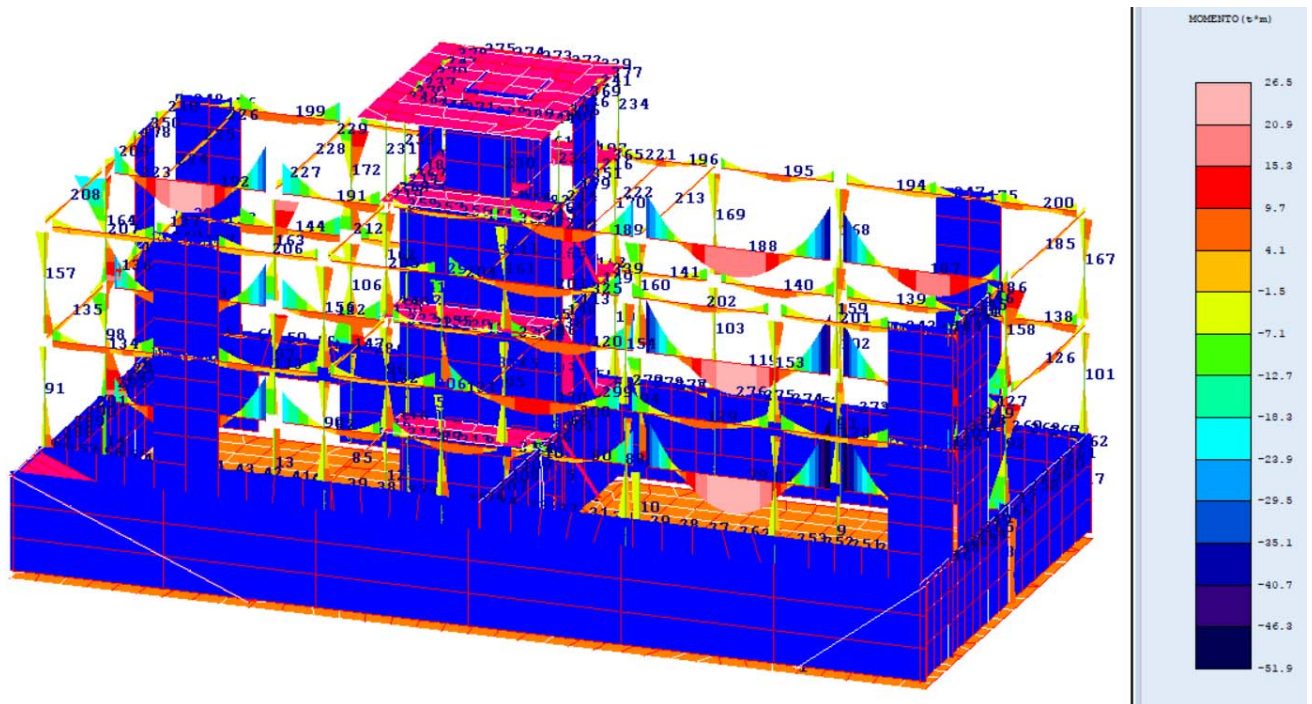
Fig.22-vista n.1_ Sforzi Momento Mx-My_involuppo_Corpo A
