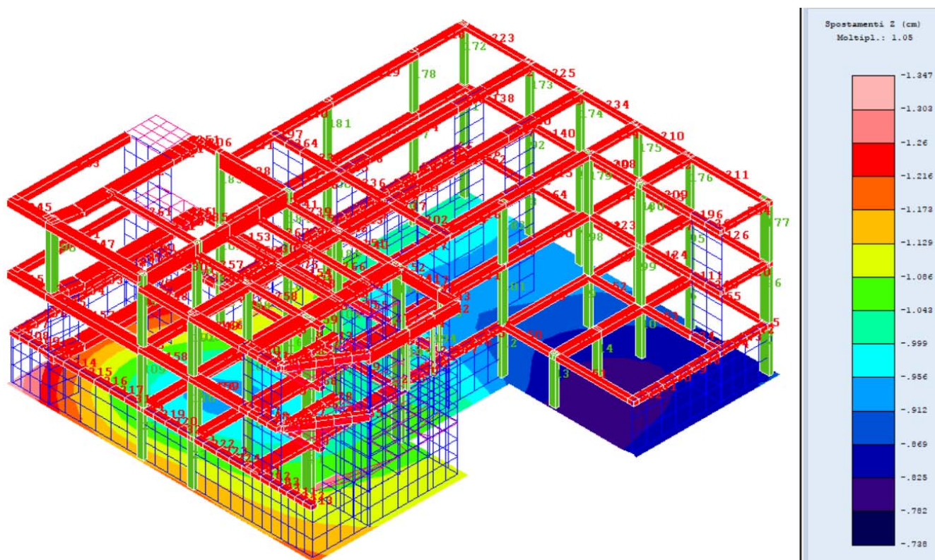
Fig.45-vista n.2_ Spostamenti z_Corpo B
