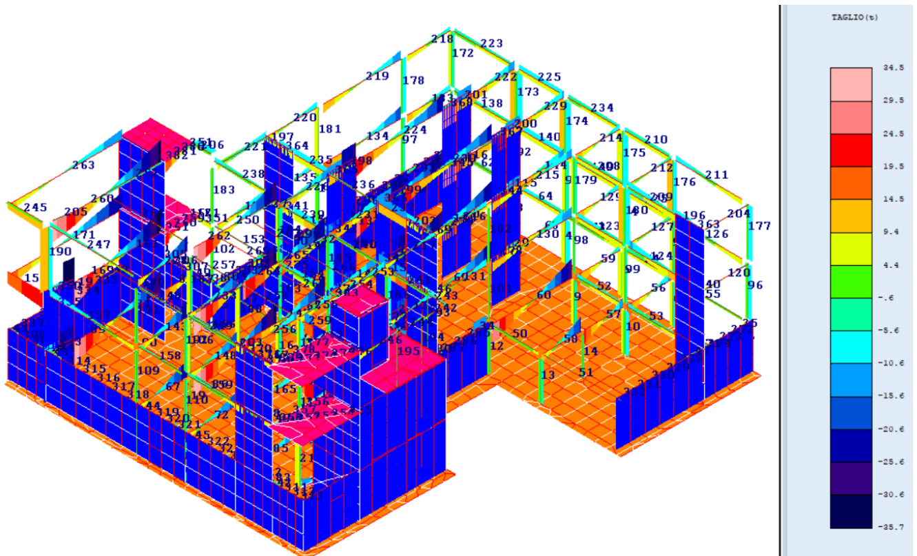
Fig.39-vista n.2_ Sforzo di Taglio Tx-Ty_involuppo _Corpo B
