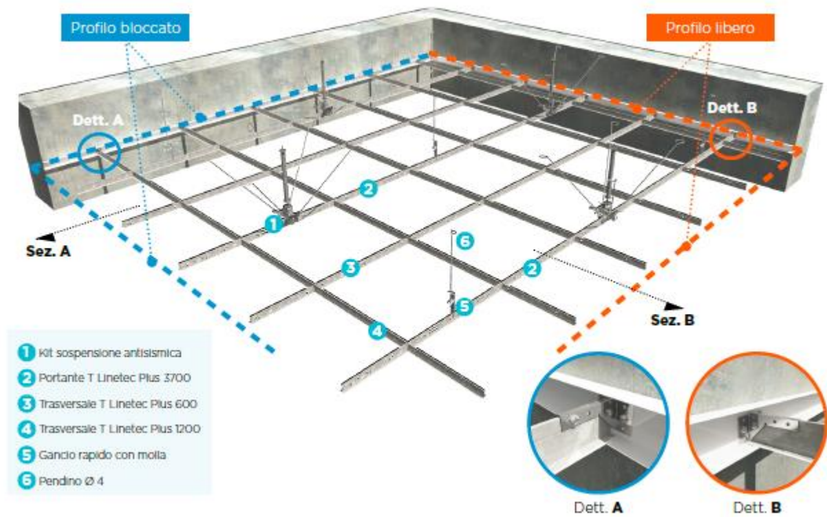
Figura 2: installazione del sistema G-Seismic Top su controsoffitto in cartongesso modulare.
