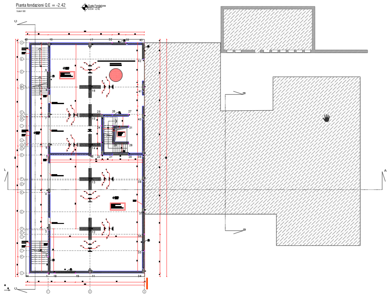
Figura 5 – Fondazioni corpo A FASE I
