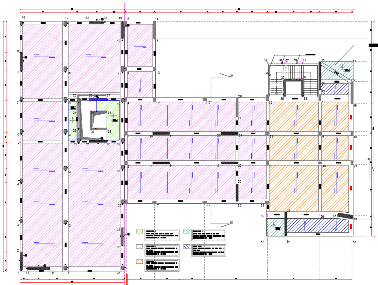
Figura 9 - Key plan 2° impalcato
