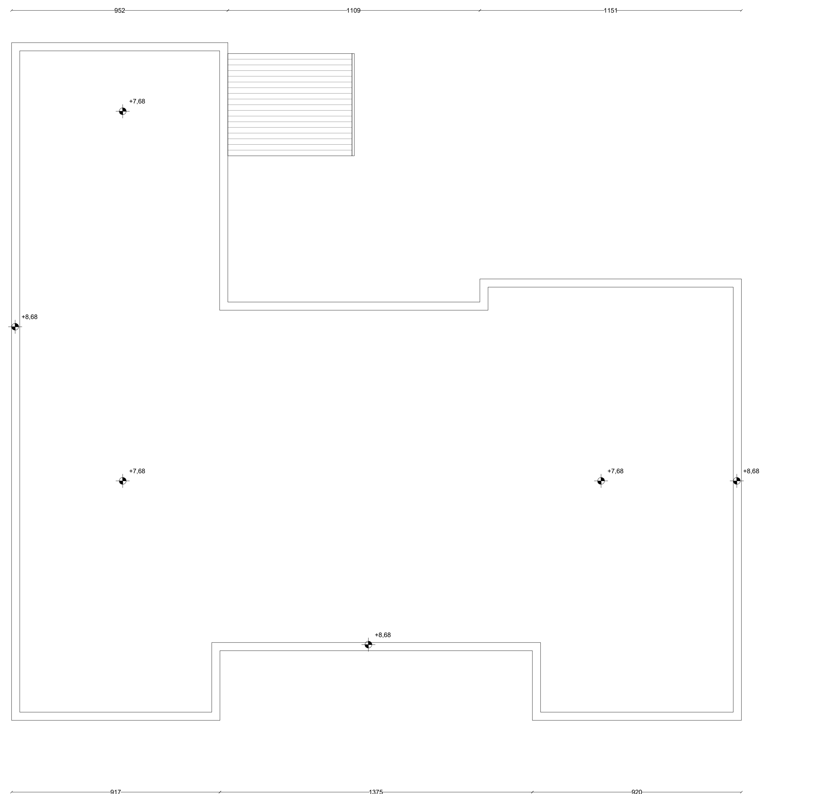
PIANO COPERTURA scala 1:100
