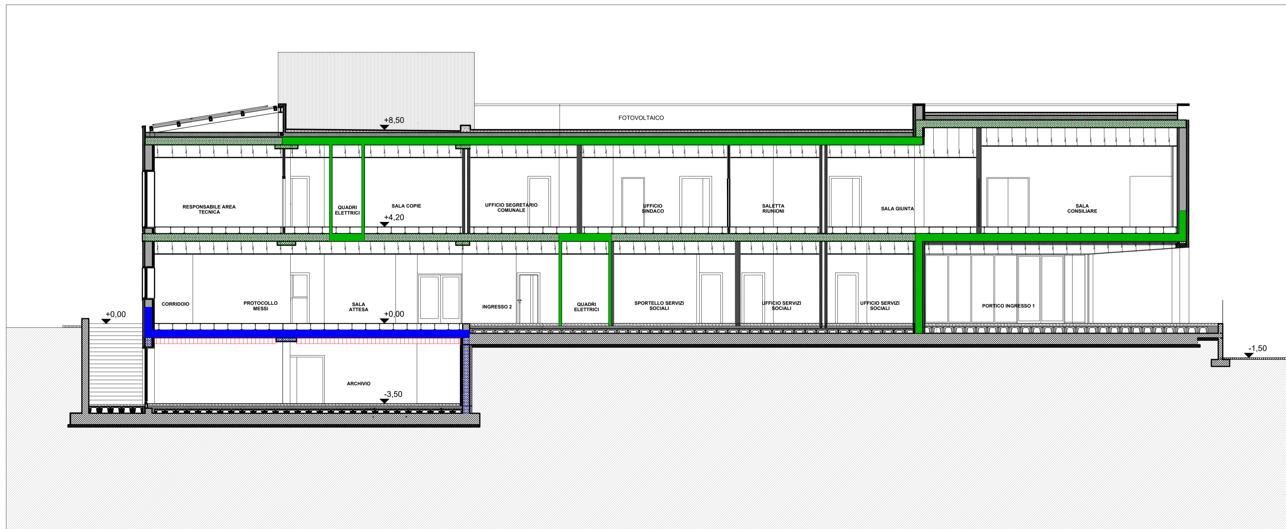
SEZIONE LONGITUDINALE
