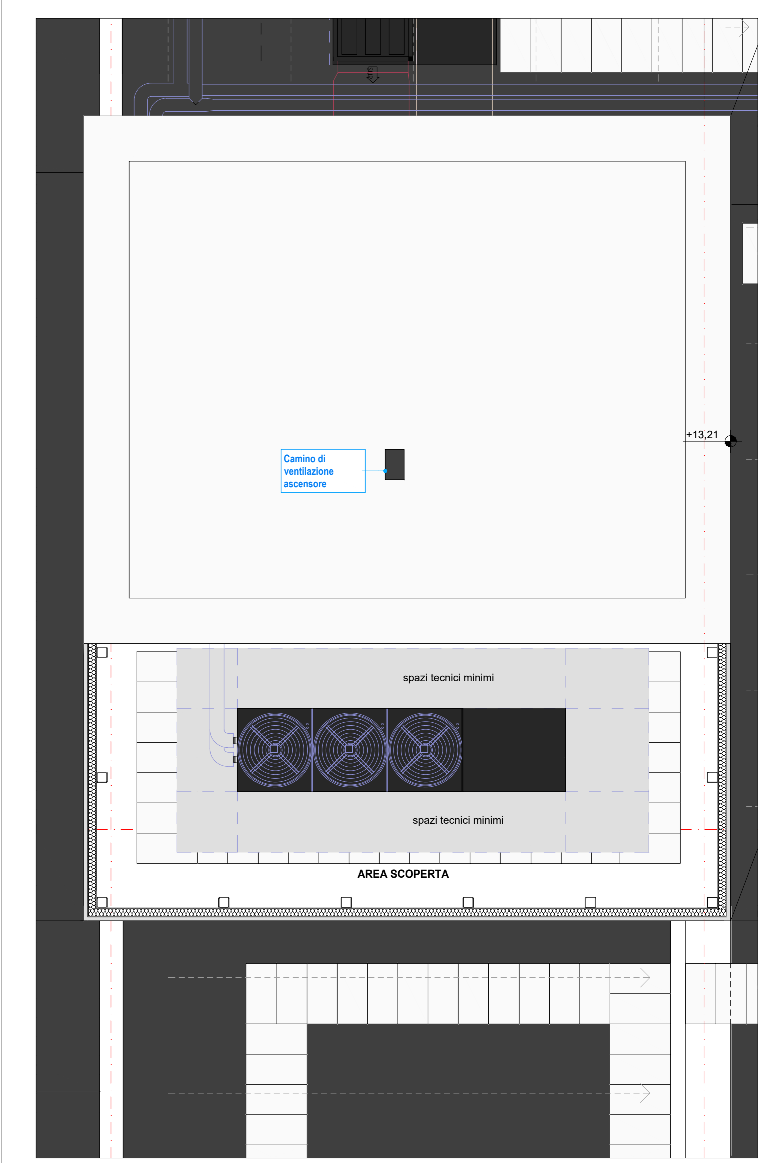
COPERTURA scala 1:50
