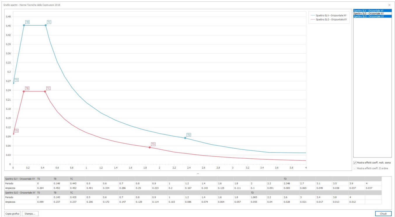
Fig. 5 – Spettri sismici
