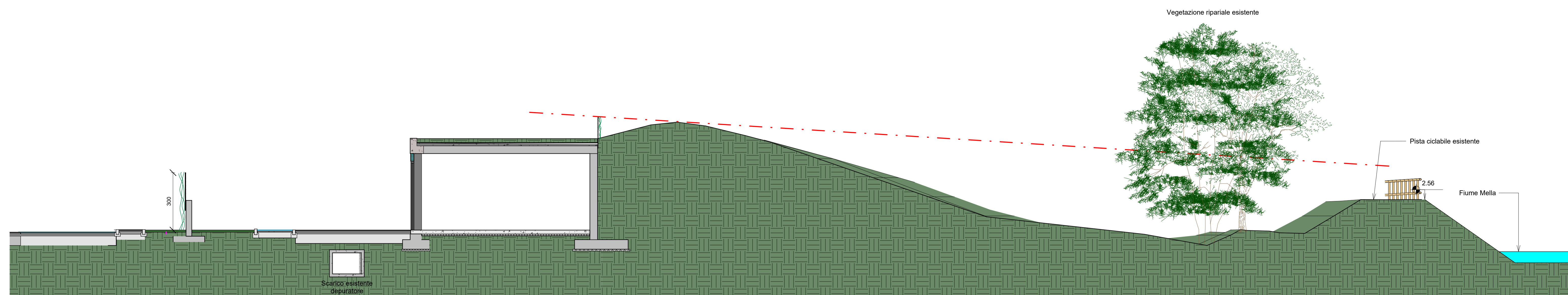
S1V01C Sezione generale 1 - Progetto VARIANTE 01 A.V. 26 1 : 100
