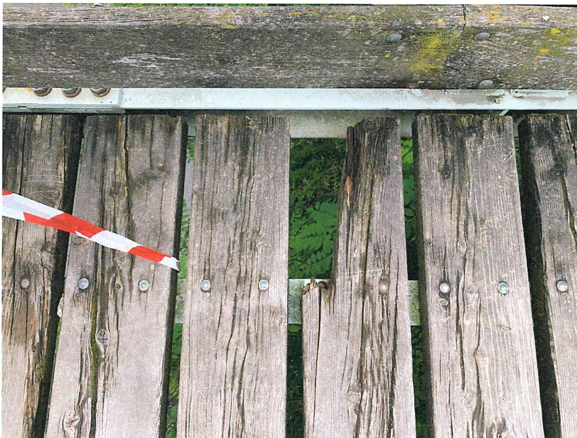
Dettagli degli elementi in legno dell'assito del ponte esistenti
